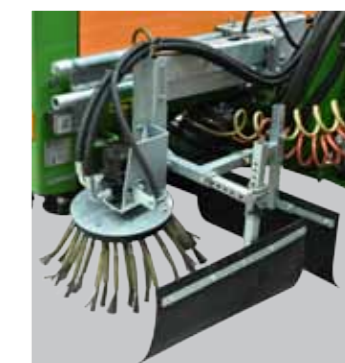
Гидравлическое управление выдвжной щеткой для очистка желобов
